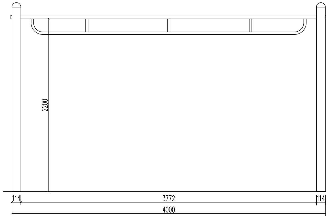
天梯立面图
